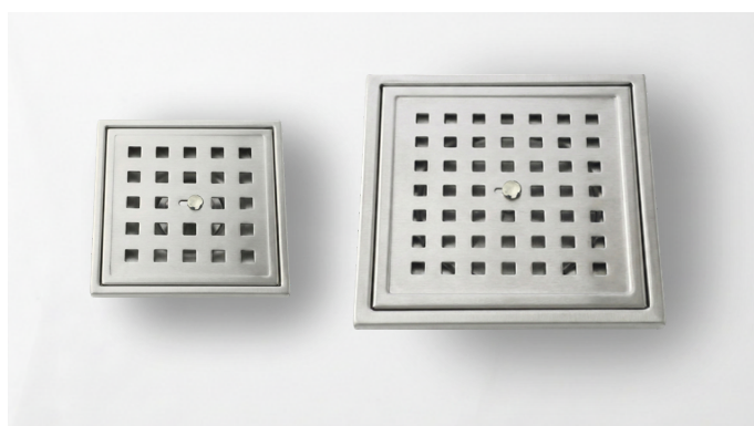
QD118AES - 10x10 / QD119AES - 15x15 SISTEMA ABRE E FECHA / AÇO ESCOVADO
